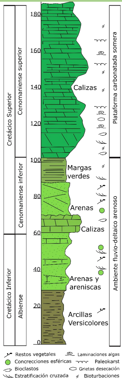
Figura 2. Serie estratigráfica del entorno de Chinchilla. Todo estos sedimentos se depositaron entre hace 113 Ma (inicio del Albense) y 94 Ma (finales del Cenomanense).
