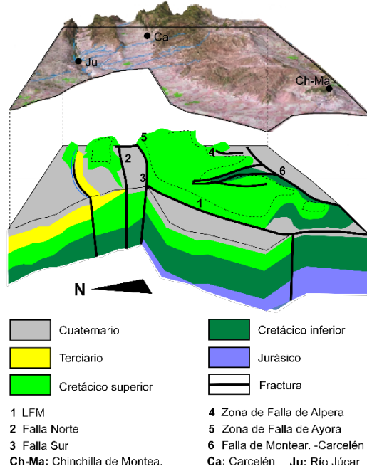
Figura 5. La Sierra Montearagón-Carcelén se haya limitada, por la Fosa de Carcelén-Ayora, al Norte, la Fosa de Alpera-Ayora al Este, la Fosa de las Rochas y la Falla de Montearagón-Alpera, al Sur, y la prolongación de la Línea de Fracturación Múltiple (LFM), al Oeste. La magnitud del desplazamiento vertical del terreno puede situarse hasta en 300 m. Figura tomada de Gómez-Alday, J. J., Castaño, S., & Sanz, D., (2007). Geología. En: La sierra de Chinchilla. El centro de adiestramiento (cenad) Chinchilla y sus condiciones ambientales. Ed: Ministerio de Defensa. ISBN: 978-84-9781-310-5.
