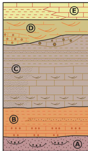
Figura 4. columna estratigráfica del Mioceno del Prebético. La unidad B no aparece en este Geolodía.
