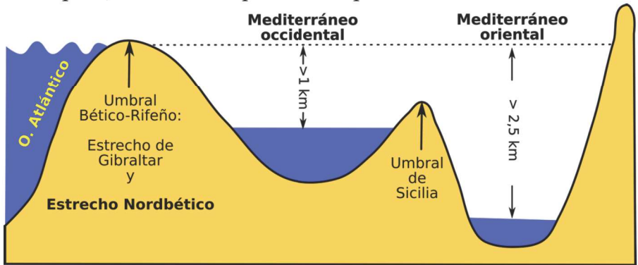
Figura 1. Nivel del agua del Mediterráneo hace 5,5 Ma. Las dos partes del Mediterráneo se desconectaron del Atlántico y entre sí, formando mares con profundidades de hasta 2,5 km.
